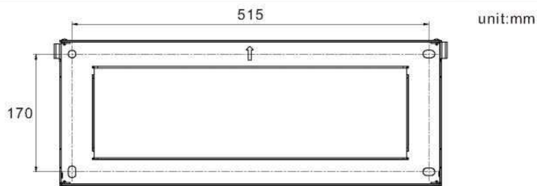
Obrázek 4.3 Montáž střídače na stěnu
