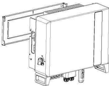
Obrázek 4.4 Nástěnná montážní konzola
